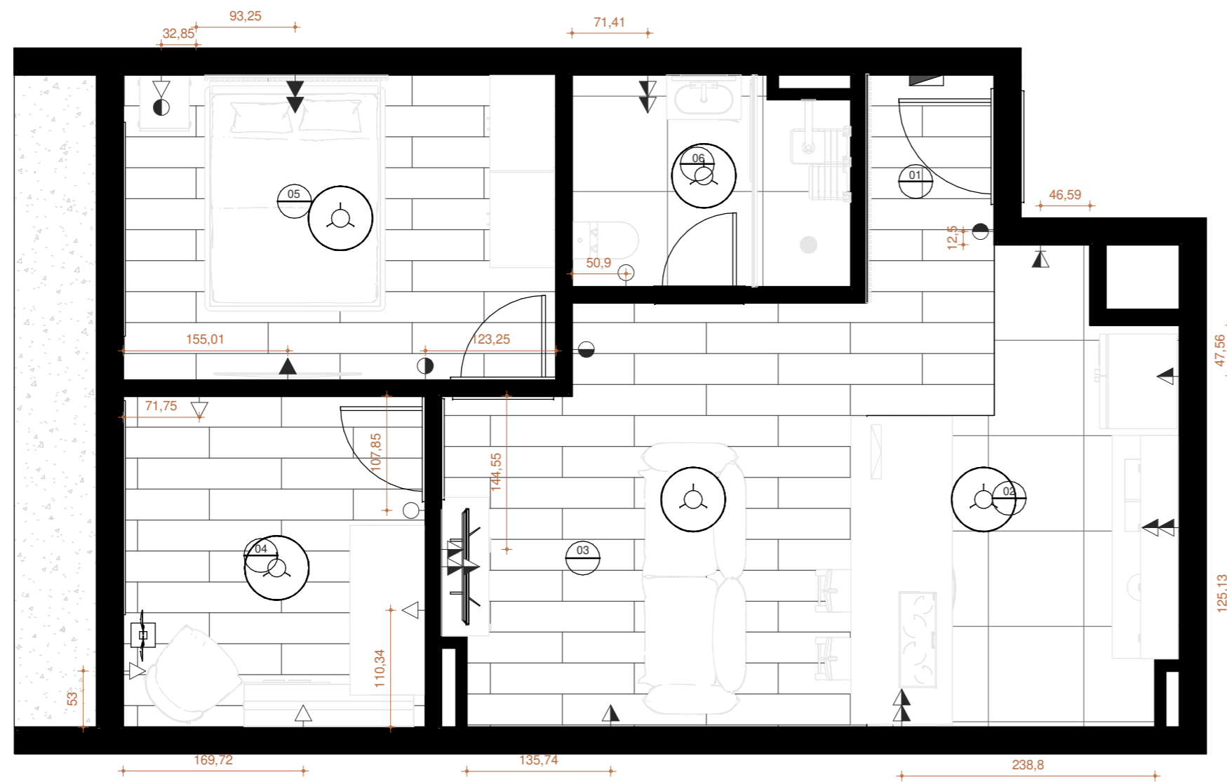
1 PLANTA BAIXA - PONTOS ELÉTRICOS
